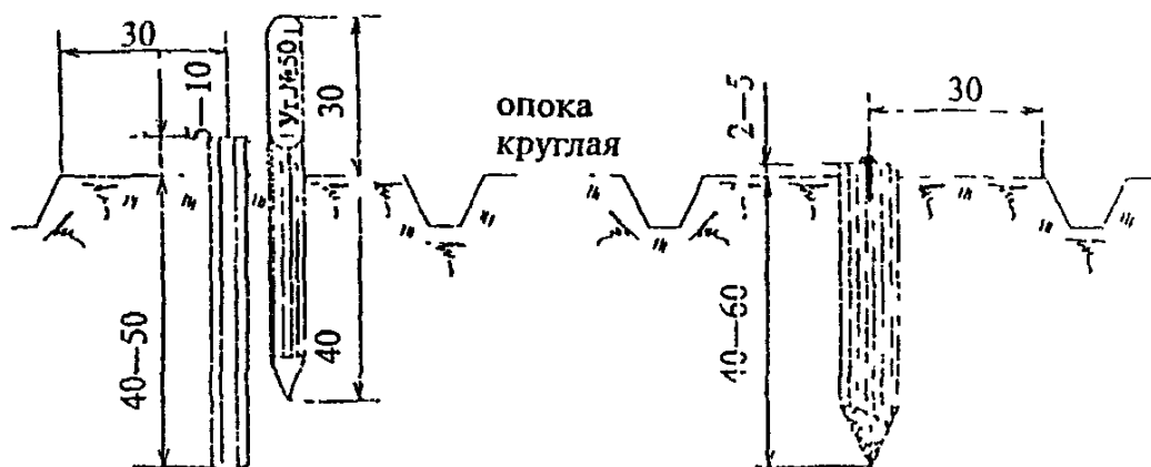
1. Металлическая труба, кованый гвоздь со стержнем
