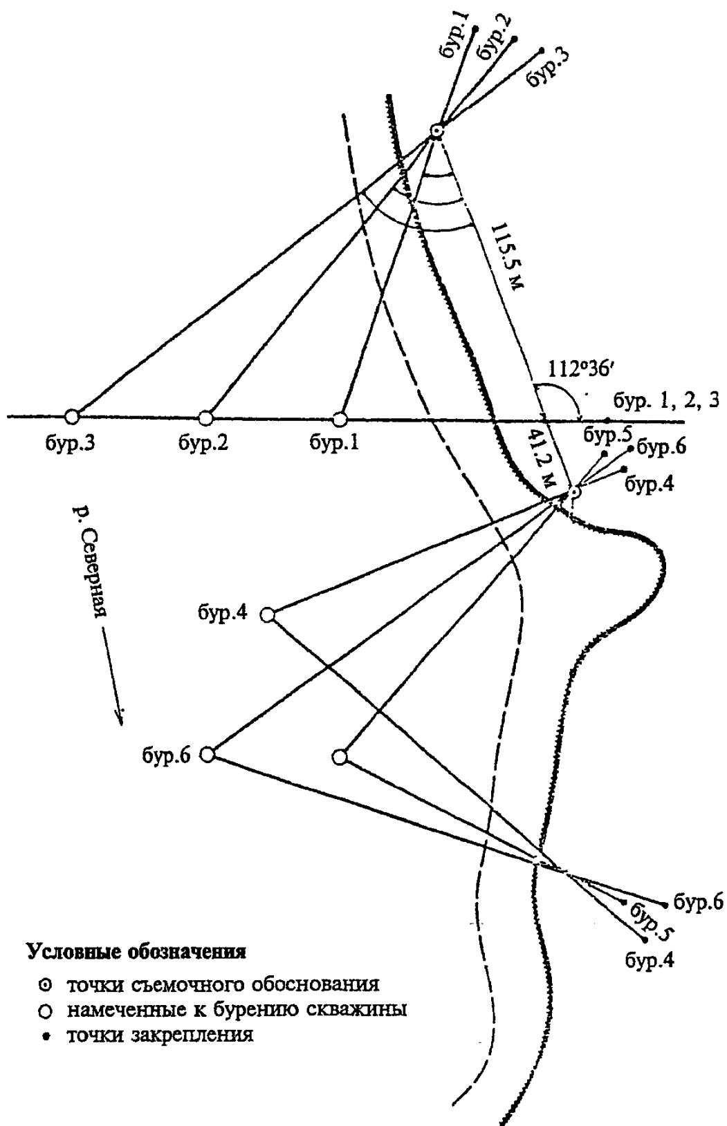
Рис. 4. Схема закрепления акватории створами вынесенных в натуру буровых
