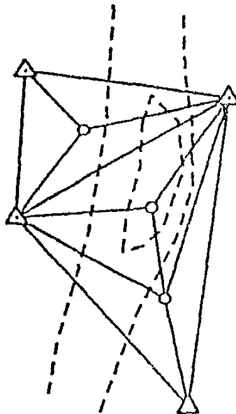
2. Цепочка треугольников и засечка
