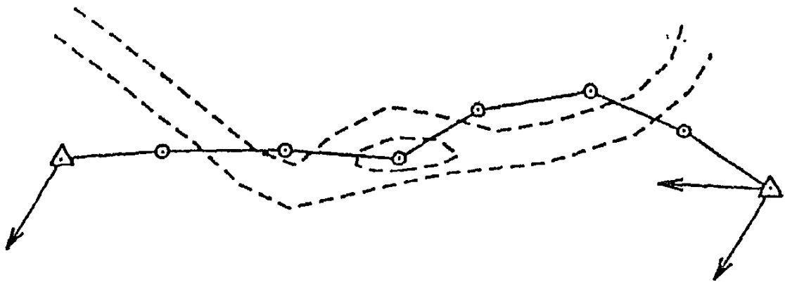
1. Одиночный полигонометрический ход
