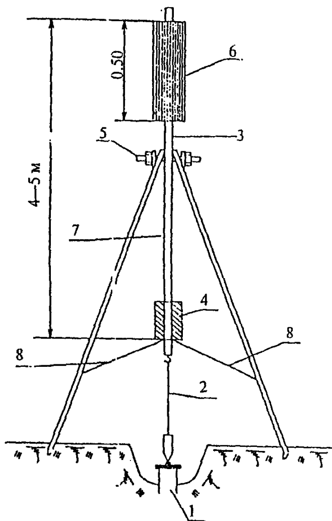
Металлическая или деревянная веха с противовесом
