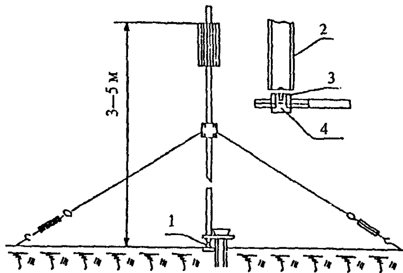
Съемная металлическая веха с визирным цилиндром
