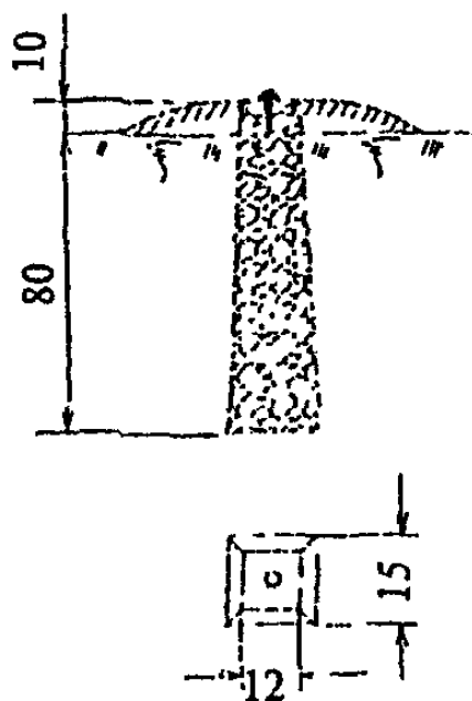
1. Бетонный пилон
