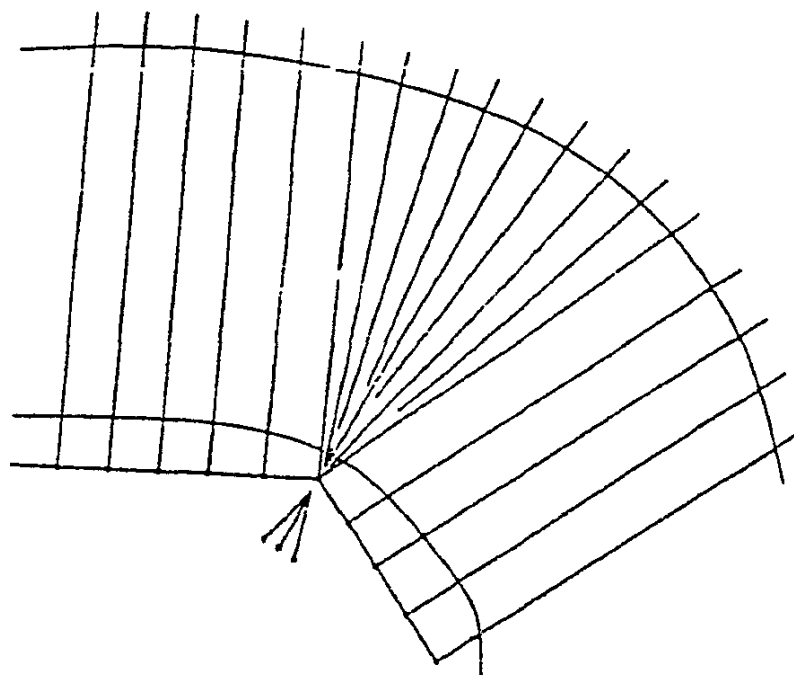
Рис. 1. Схема разбивки радиальных галсов
