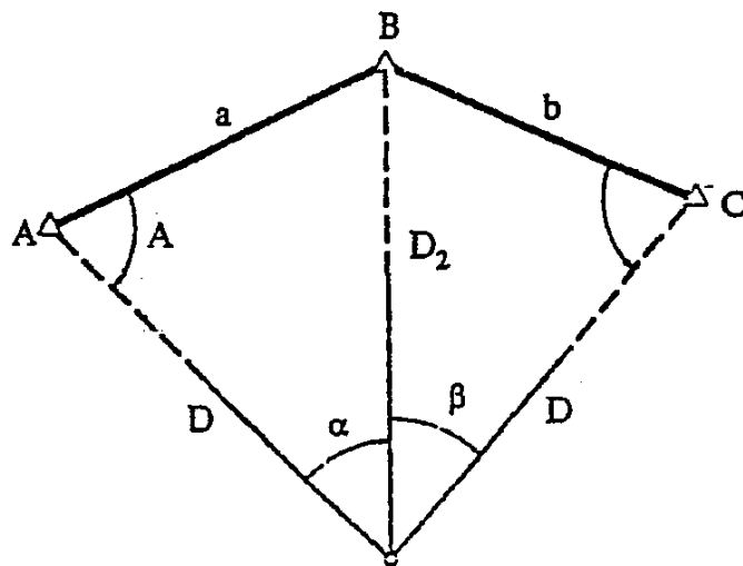
а) по трем смежным пунктам
