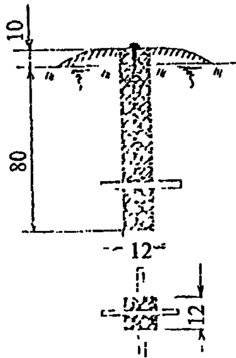
1. Бетонный пилон
